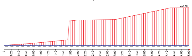
Grenzquerkräfte
