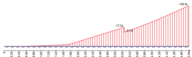
Grenzmomente
