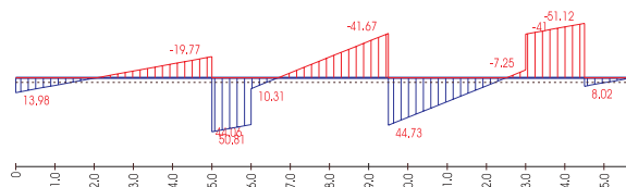
Zugehörige Grenzerkraft zum Momentenverlauf
