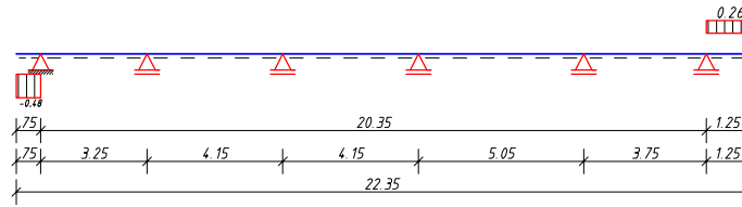
EWG 320 Wind v.li. FGF Druck (Kat. Q,W) in z-Richtung
