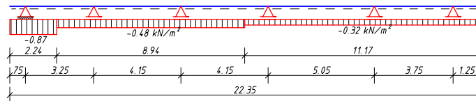
EWG 100 Ständige Einwirkungen (Kat. G) in y-Richtung
