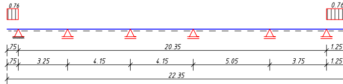
EWG 510 Wind 90/270° Unterwind (Kat. Q,W) in z-Richtung
