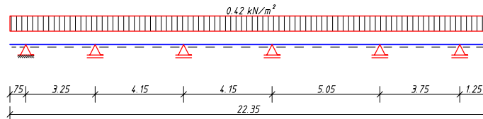
EWG 100 Ständige Einwirkungen (Kat. G) in y-Richtung
