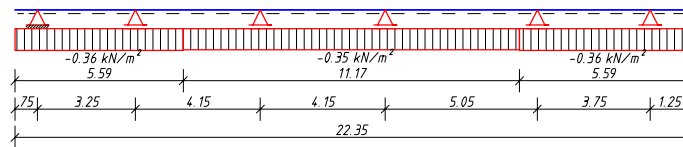
EWG 322 Wind v.li. H Druck (Kat. Q,W) in z-Richtung
