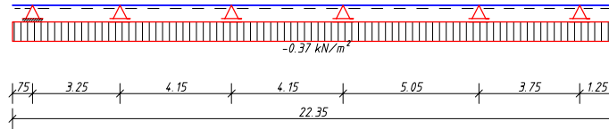
EWG 510 Wind 90/270° Unterwind (Kat. Q,W) in z-Richtung
