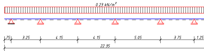
EWG 322 Wind v.li. H Druck (Kat. Q,W) in z-Richtung
