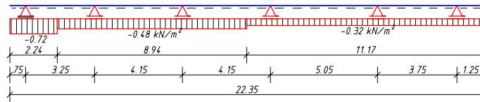
EWG 525 Wind 90° GHI Sog (Kat. Q,W) in z-Richtung
