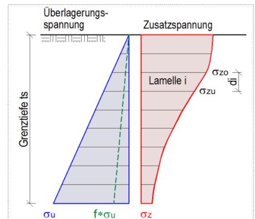
Bild 4: Spannungsberechnung
