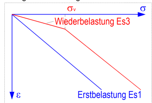
Bild 1: Linearität des Baugrundverhaltens
