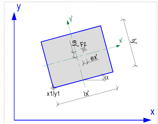
Bild 3: Koordinatensystem und Geometrie
