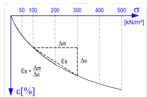
Bild 2: Nichtlineares Baugrundverhalten
